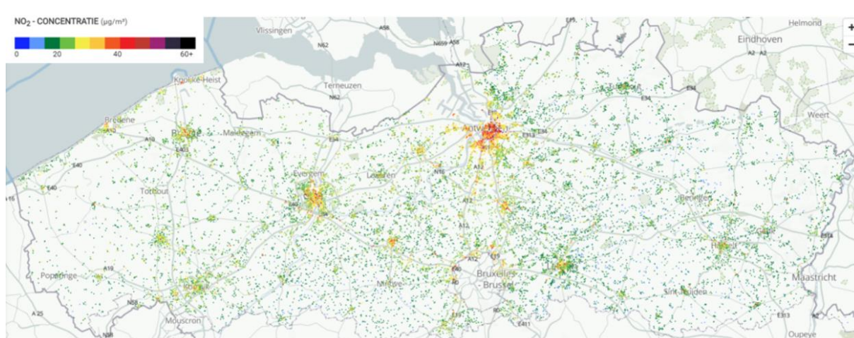
Figuur 3: Weergave van de gemeten \text{NO}_2 -concentraties met passieve samplers in de maand mei 2018, in het kader van het project Curieuzeneuzen Vlaanderen.
